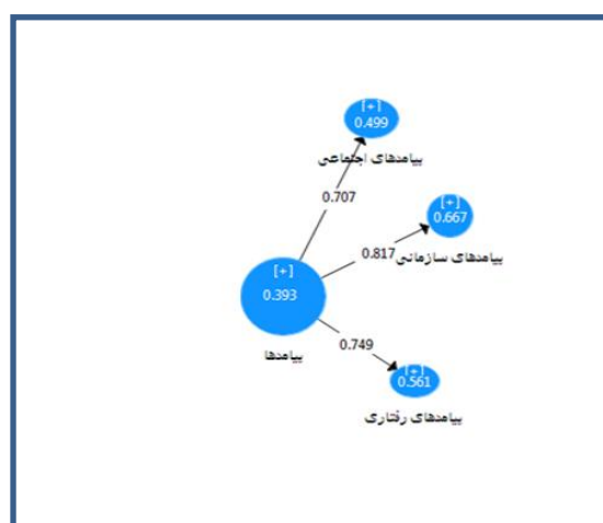
شکل ۳: مدل ساختاری تحقیق در حالت استاندارد
