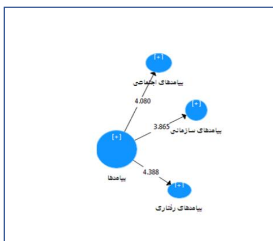
شکل ۴: مدل ساختاری تحقیق در حالت معناداری
